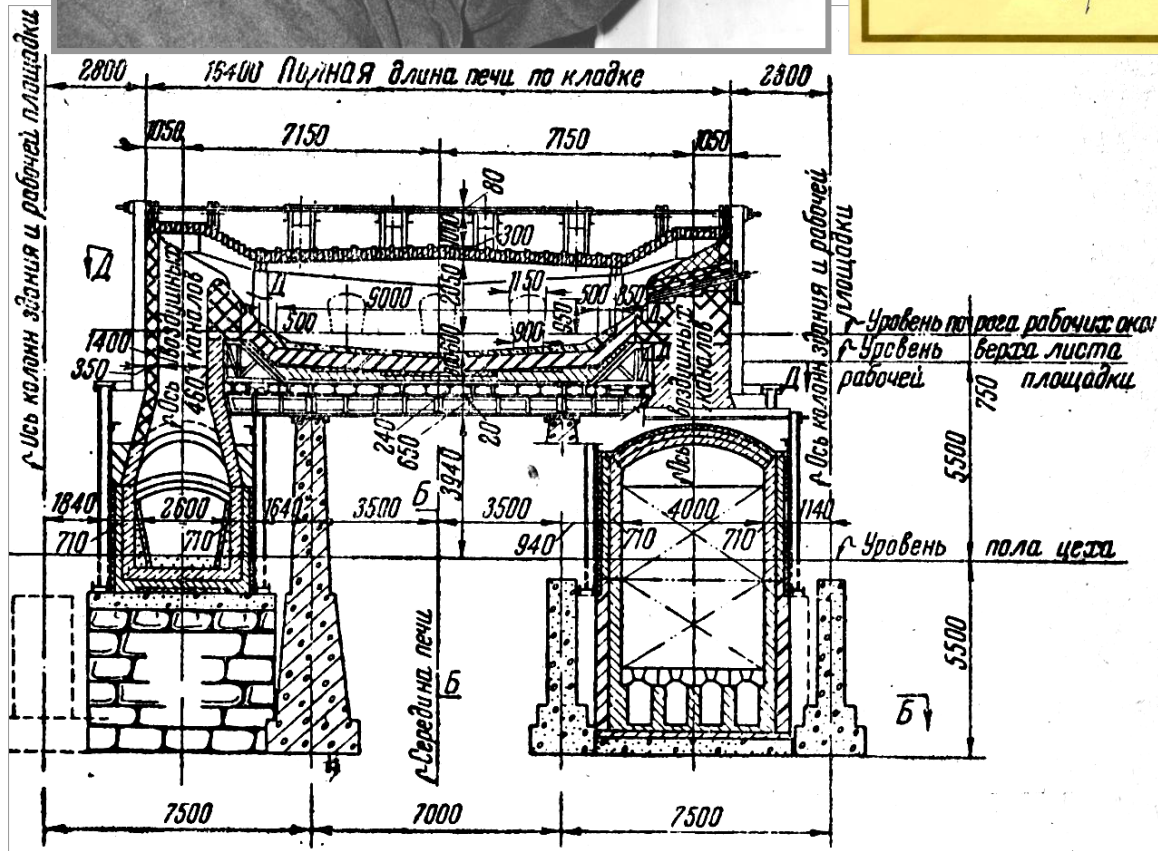
Разрез 185-т мартеновской печи. К курсовому проекту автора обзора. ВМТ 1949 г.
